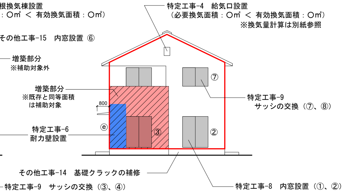
南立面図
