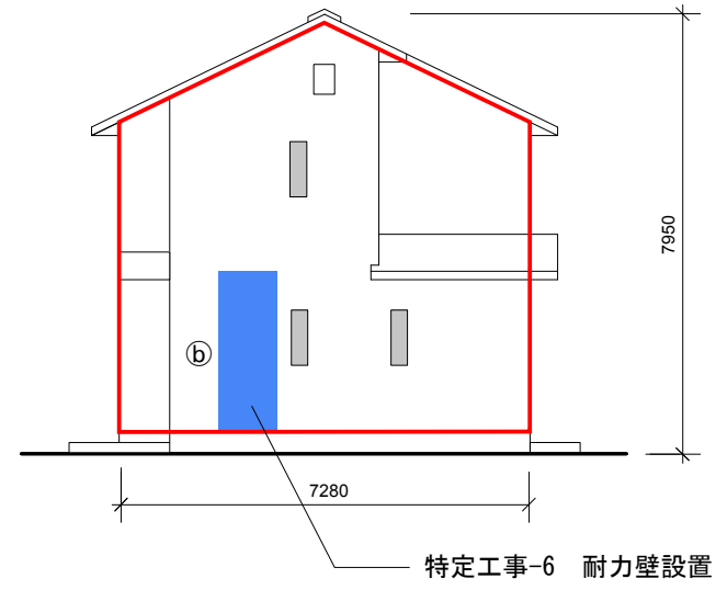
北立面図
