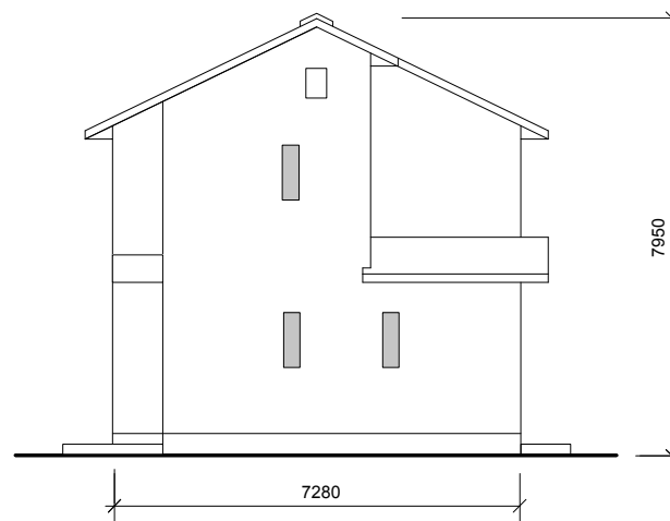
北立面図
