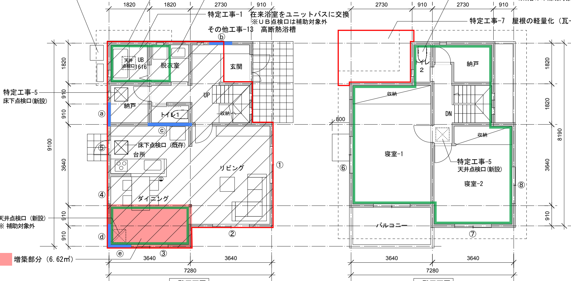
1階平面図
