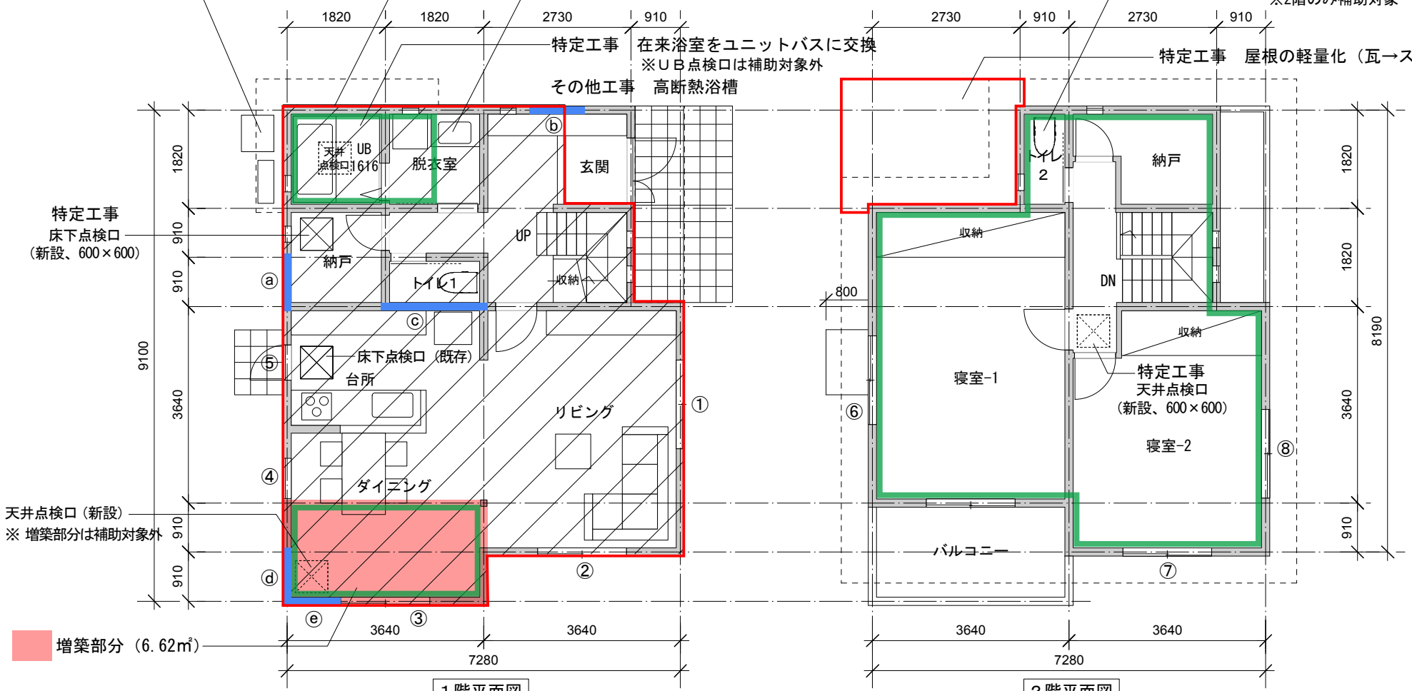
1階平面図
