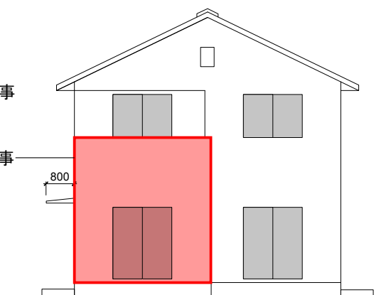
南立面図
