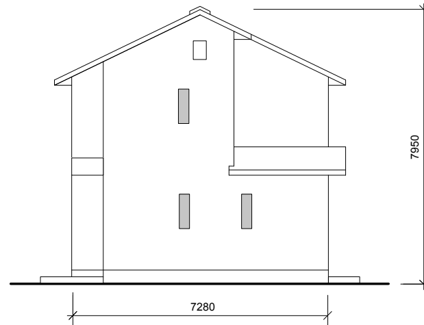
北立面図
