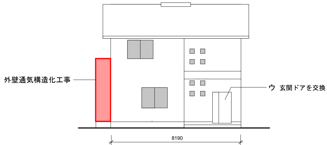
東立面図
